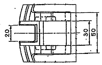
蓋裏閉蓋取付部詳細
