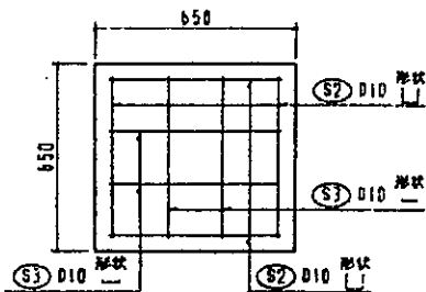
本体底版配筋図
