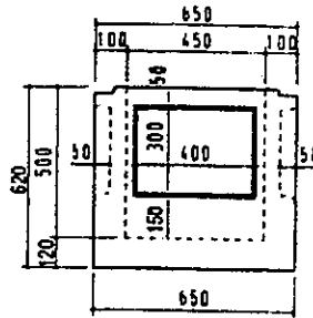
本体材形状図
