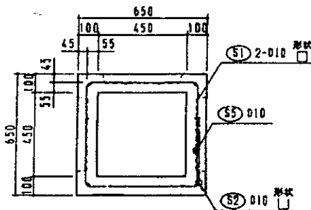
本体b-b断面配筋図
