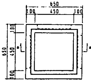
本体平面図
