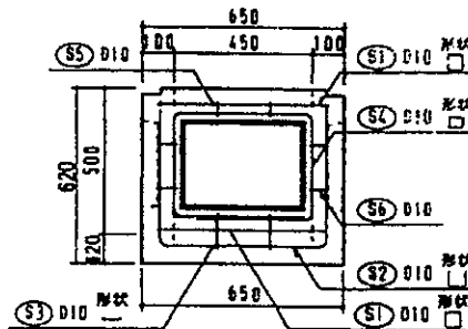
本体立面配筋図
