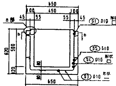
本体a-a断面配筋図
