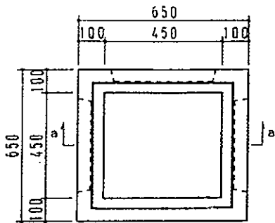
本体平面図
