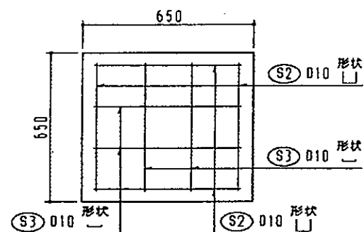
本体底版配筋図
