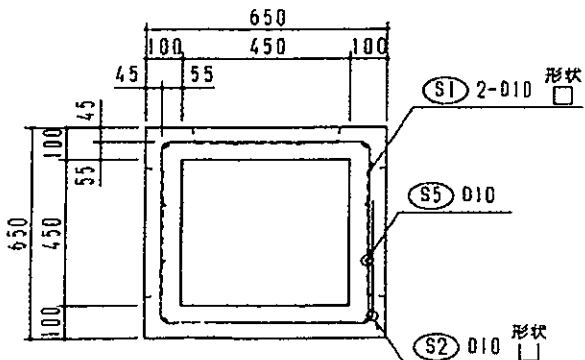
本体b-b断面配筋図
