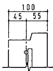
a部詳細図
