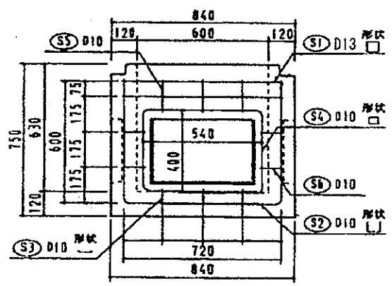
本体部材立面配筋図
