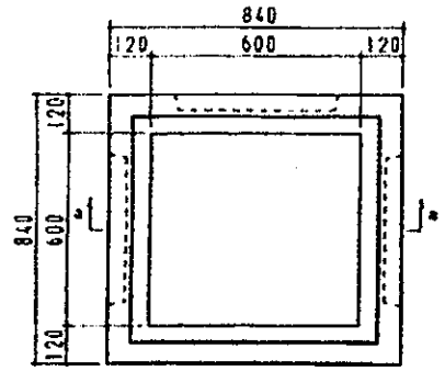
本体部材平面図
