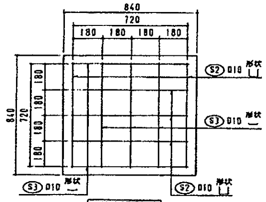
本体産版配筋図
