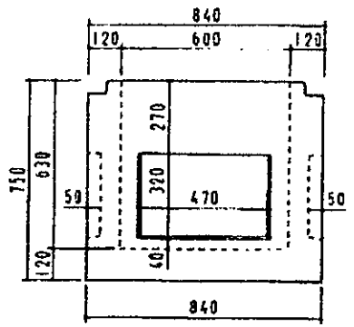
本体部材形状図
