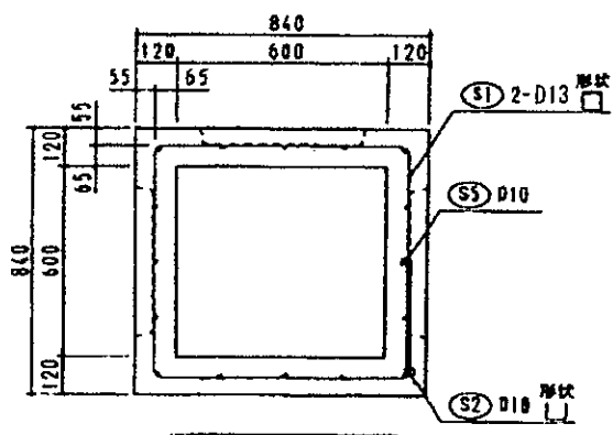
本体 b-b 断面配筋図
