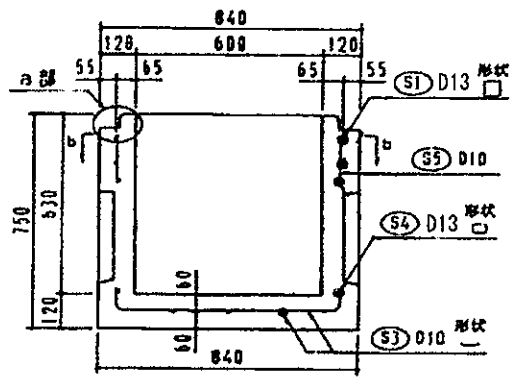
本体部材 a-a 断面配筋図
