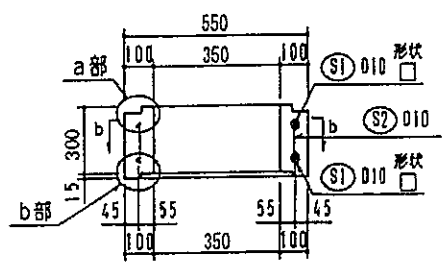
本体a-a断面配筋図
