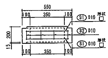
本体立面配筋図
