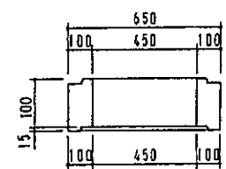
本体a-a断面図
