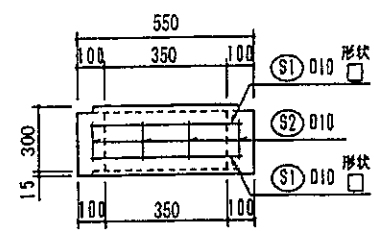
本体立面配筋図
