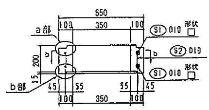
本体a-a断面配筋図
