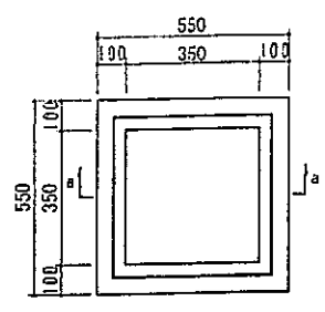
本体平面図
