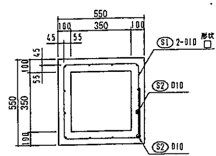
本体b-b断面配筋図
