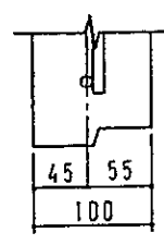
b部詳細図
