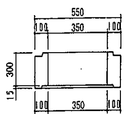
本体a-a断面図
