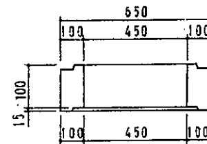
本体a-a断面図
