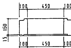
本体a-a断面図
