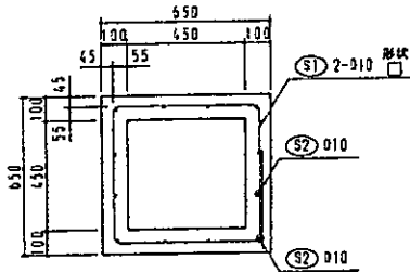
本体b-b断面配筋図
