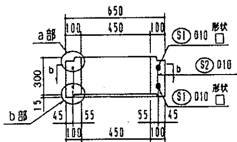
本体a-a断面配筋図
