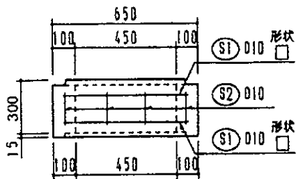
本体立面配筋図
