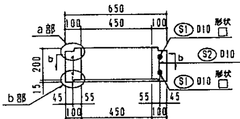
本体a-a断面配筋図
