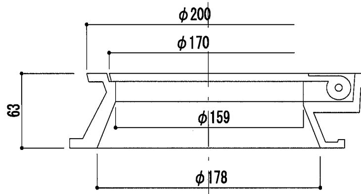
A-A' 断面
