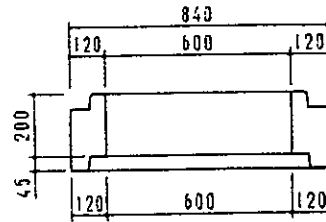
a-a断面図
