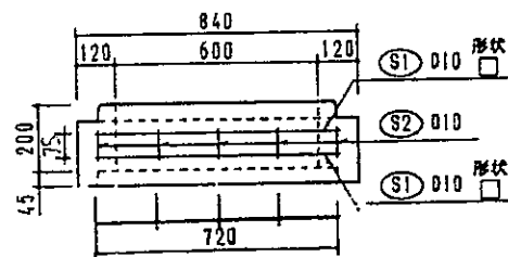
立面配筋図
