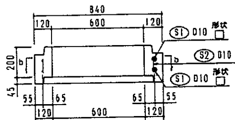
a-a断面配筋図
