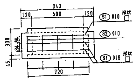
立面配筋図
