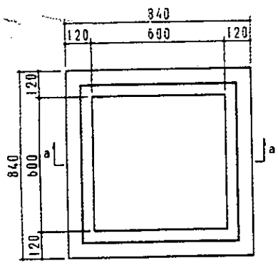
平面図
