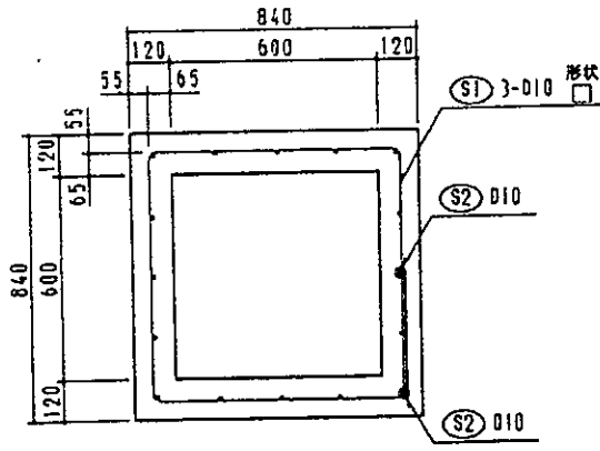
b-b 断面配筋図
