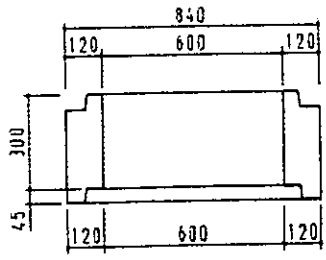
a-a 断面図
