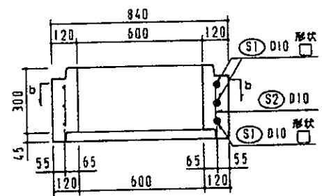
a-a 断面配筋図
